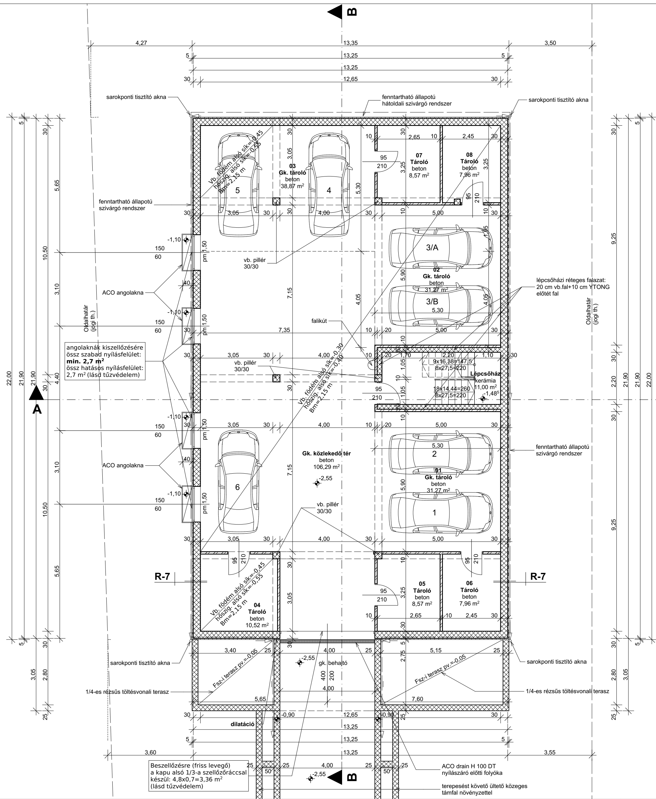
PINCE ALAPRAJZ M = 1:100
